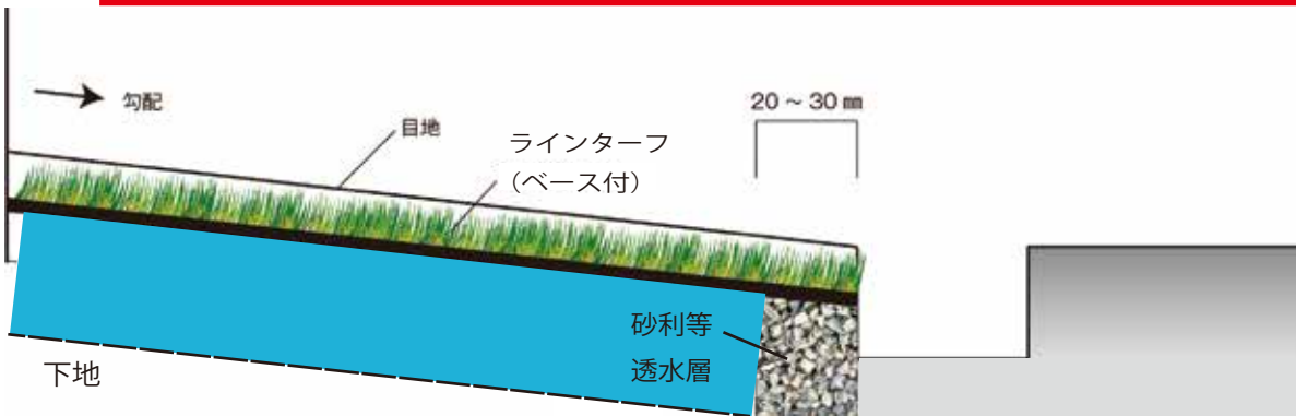
【施工断面図】
